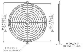
15CM二脚网罩
