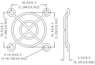
4CM网罩
