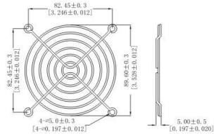
9CM网罩
