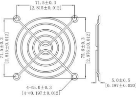
8CM网罩
