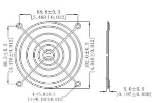
11CM网罩
