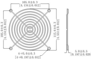
12CM网罩
