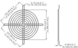
15CM四脚网罩
