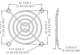
7CM网罩
