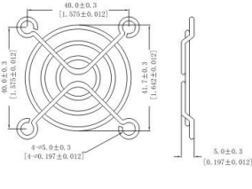
5CM网罩
