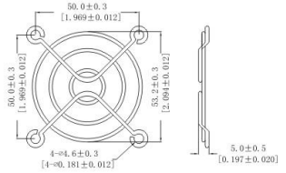
6CM网罩
